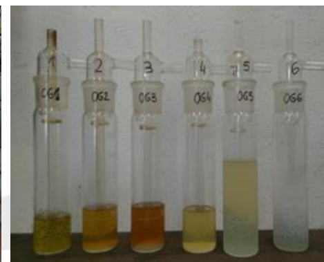
Muestreo de alquitranes CEN/TS 15439:2006
